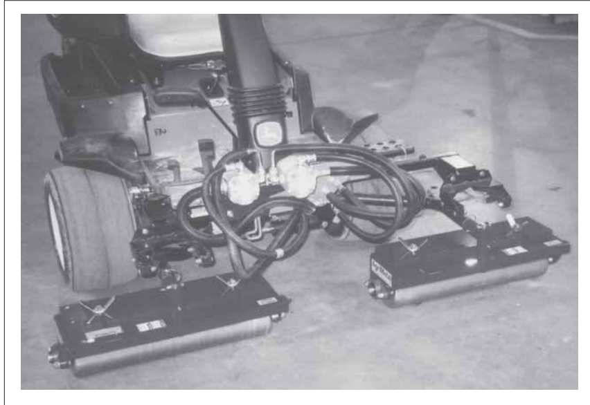
Fig. 15 MACHINE
